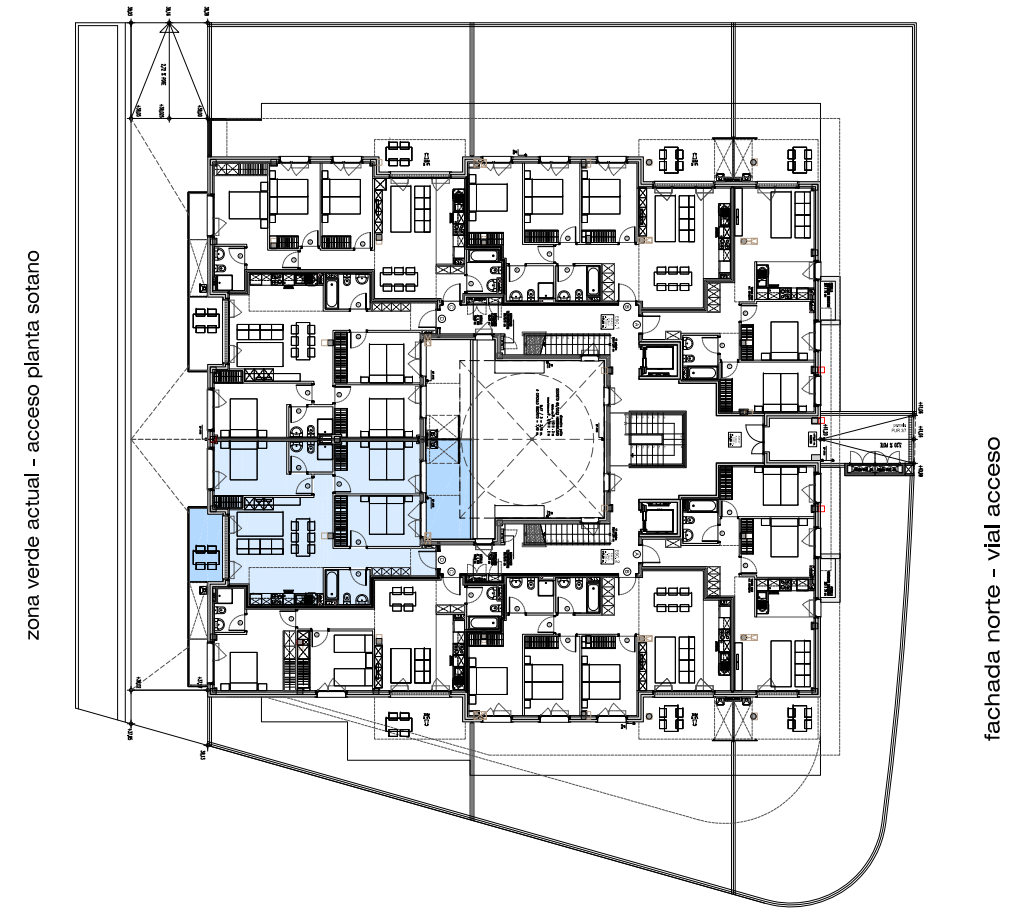
vial acceso garajes
